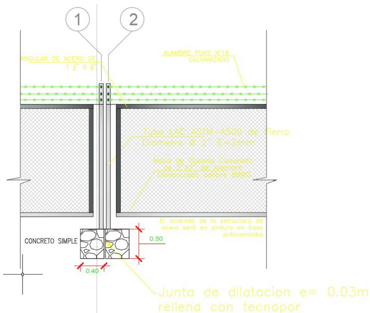
DETALLE DE JUNTA DE DILATACIÓN
