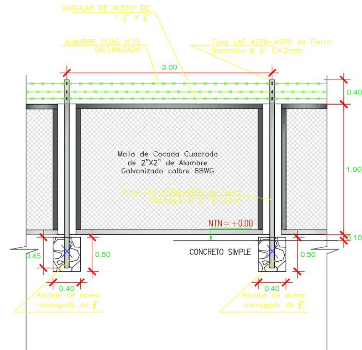
ELEVACION DE CERCO PERIMETRICO TIPO 1
