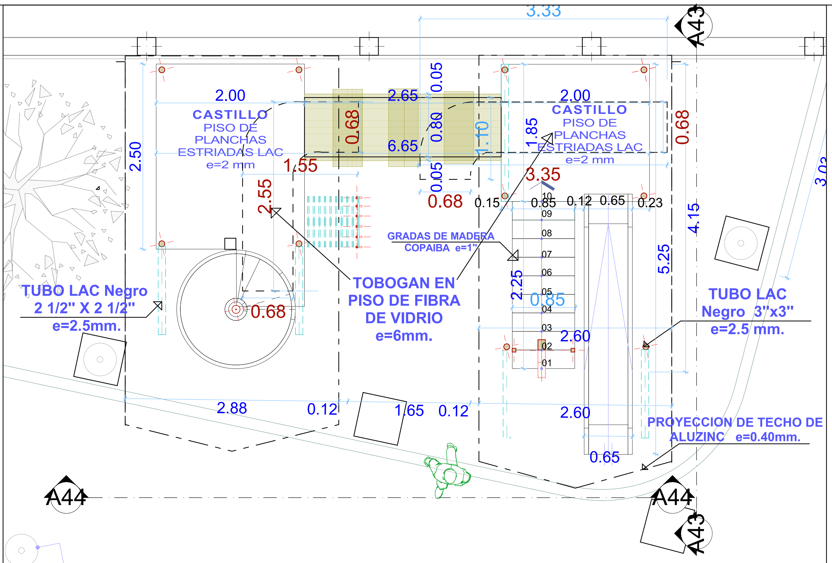
PLANO DE PLANTA DE JUEGO INFANTIL
