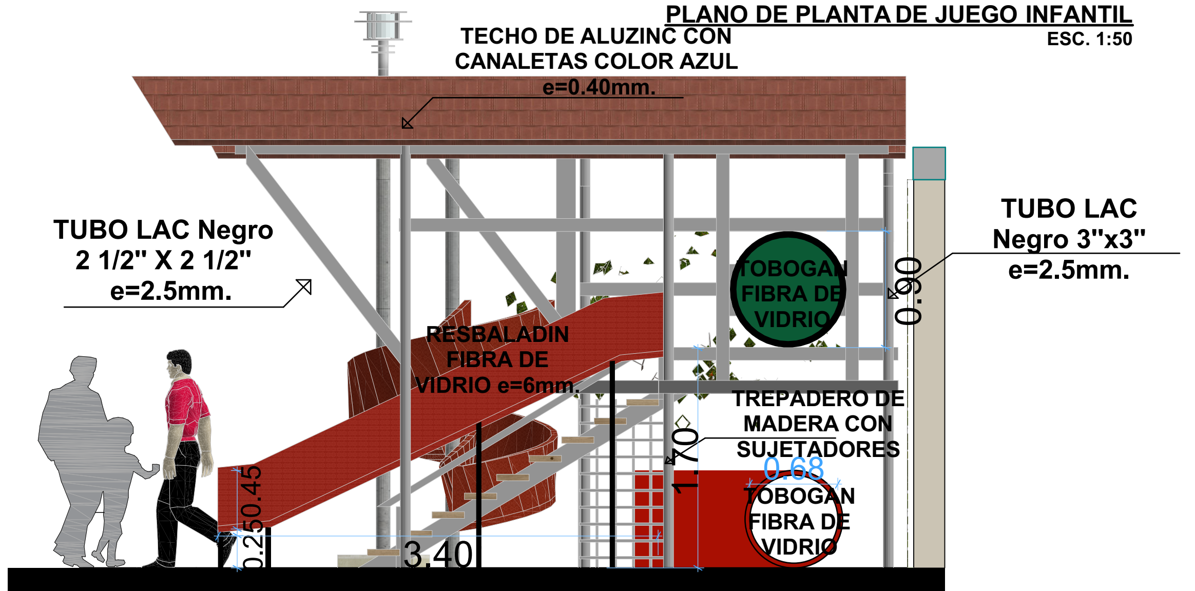
PLANO DE ELEVACION TRANSVERSAL DE JUEGO INFANTIL
